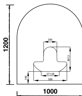
B3 en verre 6 mm d'épaisseur, raccordement dessous
