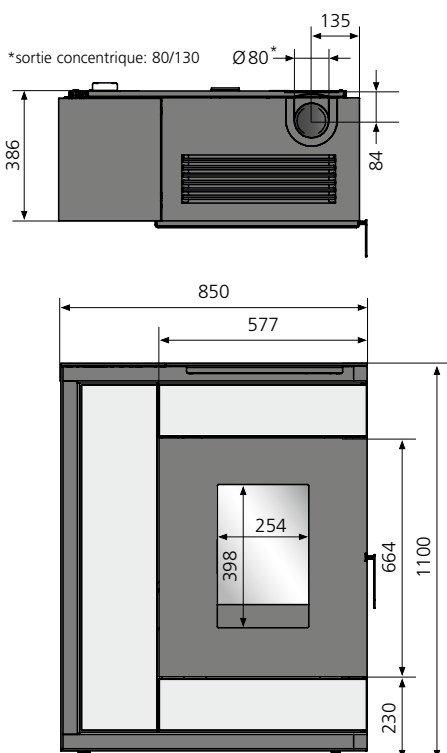
Te à piquage concentrique pour sortie par le dessus – élément prémonté de série
