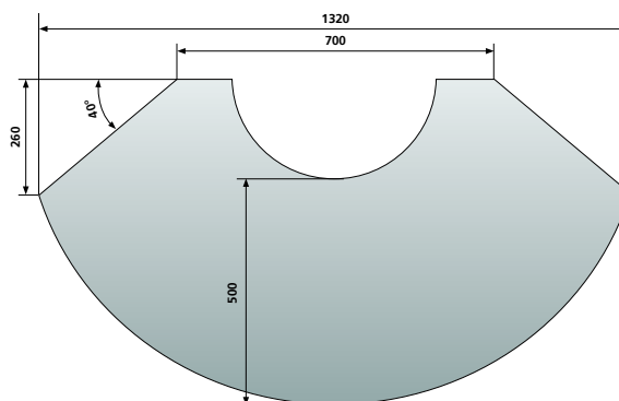
Plaque de sol avant, petit 1320 x 500 mm
